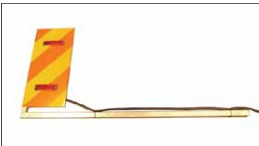
Art. nr 498114 Bred lastmarkering venstre bagerst. Komplet med rødt lys og stik.
